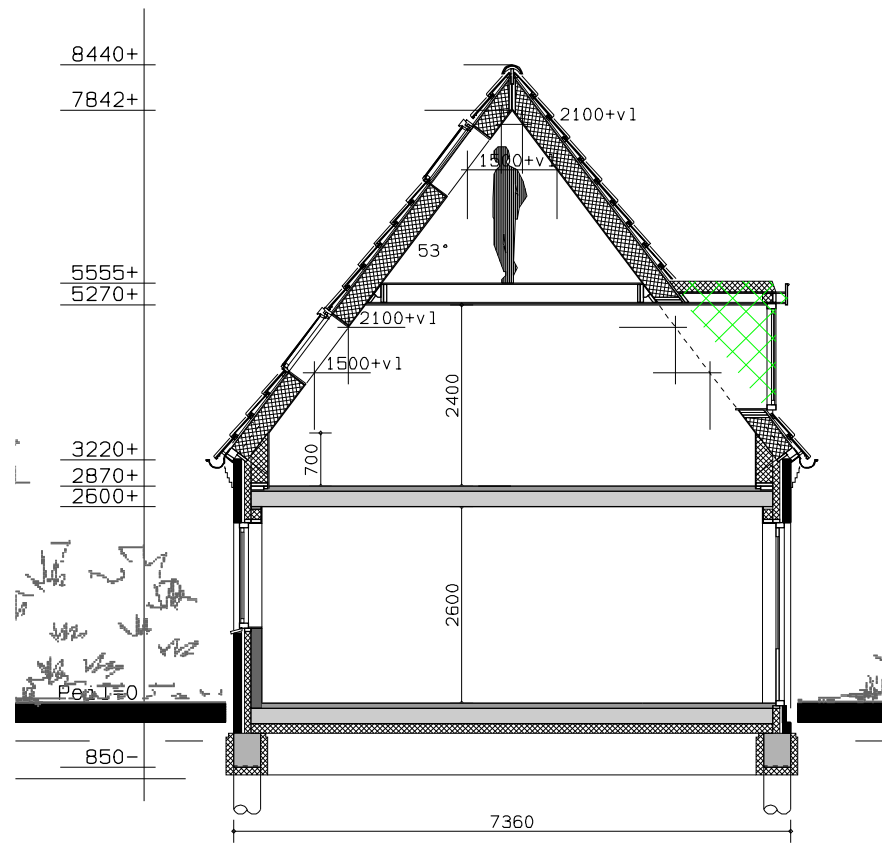
DWARSDOORSNEDE
