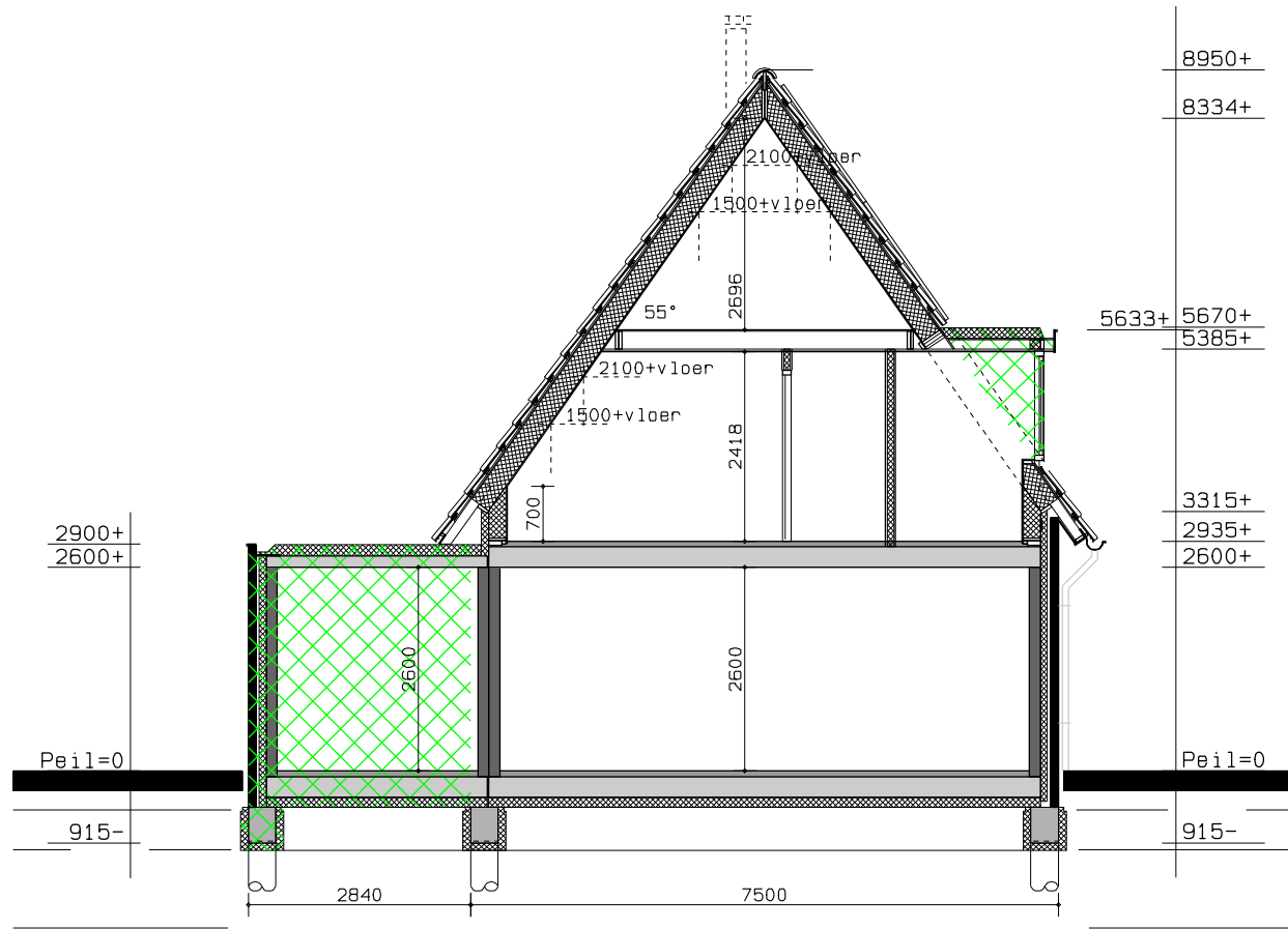
DWARSDOORSNEDE
