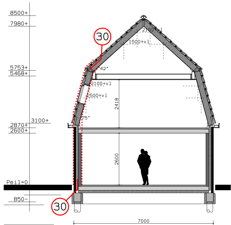
DWARSDOORSNEDE
